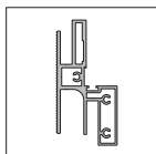
31-1322 AL31 DOOR FRAME 5300 MM AN, CM
