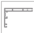
31-1607 AL31 DOOR FRAME CASING 70, 5300 MM AN, CM
