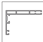
31-1607 AL31 DOOR FRAME CASING 70, 5300 MM AN, CM
