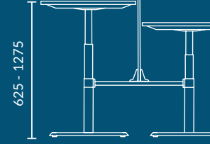
Lano-E 300 T
